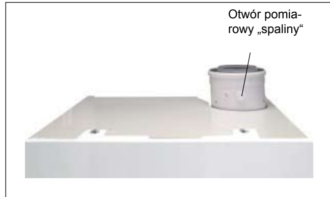
Ilustracja: Pomiar spalin przy zamkniętym urządzeniu
