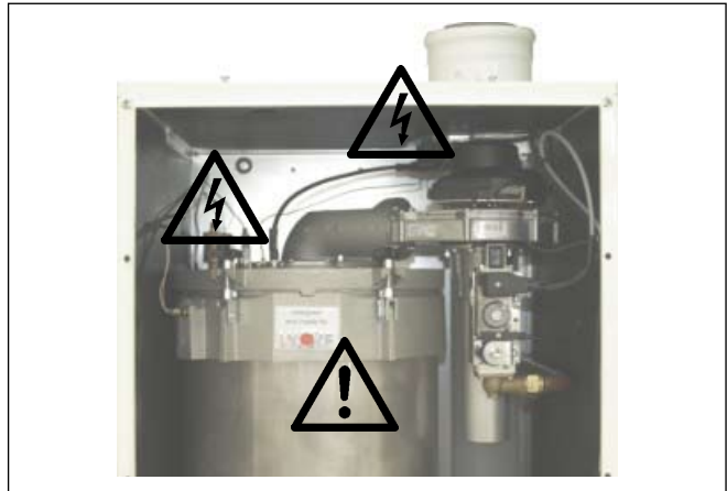
Figura: Transformador de ignición, electrodo de encendido, intercambiador de calor Peligro por tensión eléctrica, peligro de quemaduras por componentes muy calientes
