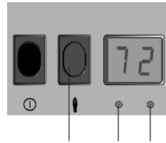
Entstörtaste Programmiertasten (-) (+)
