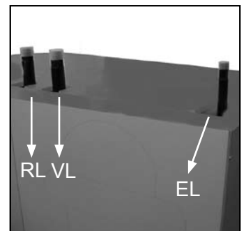
Abb. 11 BPH15 Rücklauf / Vorlauf / Entlüftung
