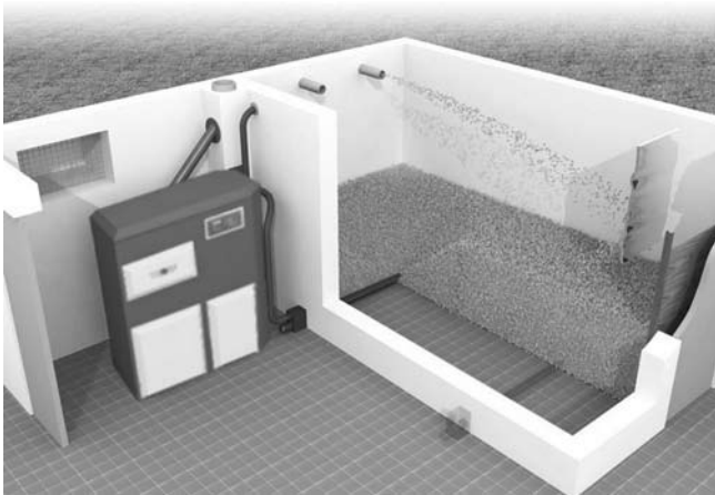
Saugsystem *
