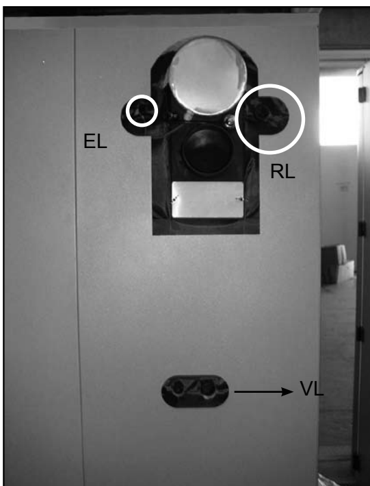
Abb. 12 BPH25/BPH35: Rücklauf / Vorlauf / Entlüftung (Bei 35kW entspricht das Saugzuggebläse nicht der Abb.)
