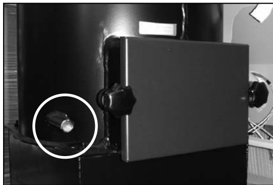
Abb. 07 Befüll- / Entleeranschluss BPH15, Anschluss 1/2 Zoll für KFE Hahn
