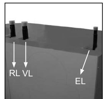
Abb. 13 BPH15 Rücklauf / Vorlauf / Entlüftung
