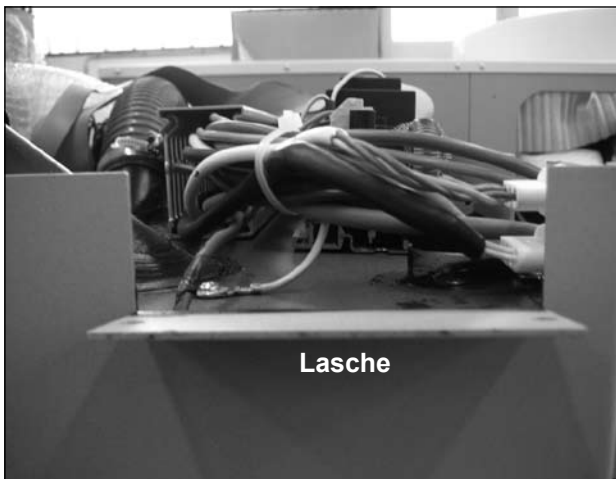
Abb. 46 Nach außen gebogene Lasche, Durchführung für Zuleitungen (Pumpem etc.)
