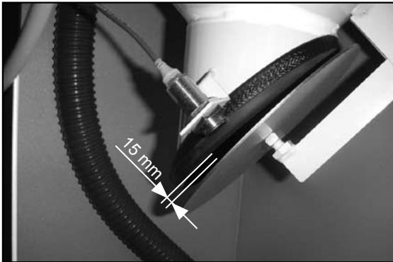
Abb. 28 Klappe offen Abstand Klappe-Dichtung , überprüfen und gegebenenfalls durch Verschieben des Gegengewichts Abstand auf 15 mm einstellen
