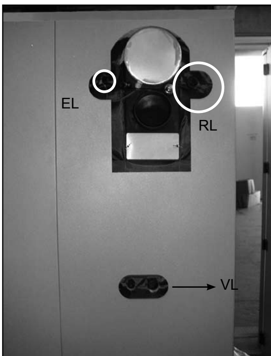
Abb. 14 BPH25/BPH35: Rücklauf / Vorlauf / Entlüftung (Bei 35kW entspricht das Saugzuggebläse nicht der Abb.)
