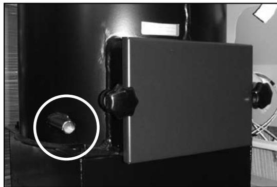
Abb. 09: Befüll- / Entleeranschluss BPH15, Anschluss 1/2 Zoll für KFE Hahn
