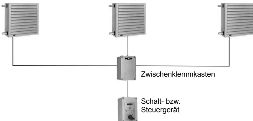
Anschluss von 3 LH-Geräten mit Zwischenklemmkasten
