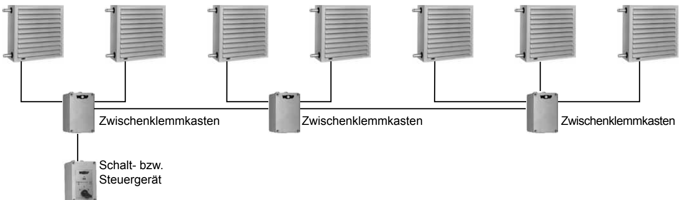
Anschluss von 7 LH-Geräten mit 3 Zwischenklemmkästen
